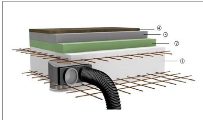
① Betondecke ② Trittschalldämmung ③ Estrich ④ Bodenbelag
