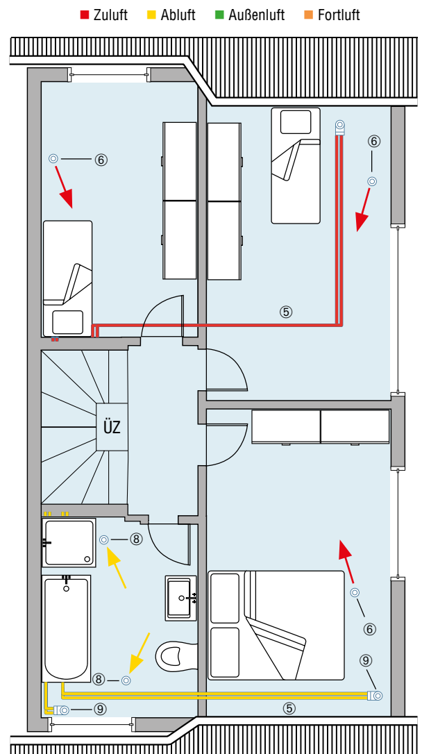
Obergeschoss
