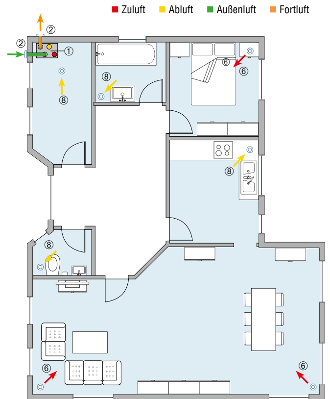
Erdgeschoss
