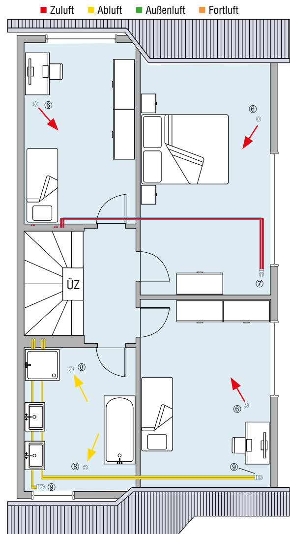
Obergeschoss
