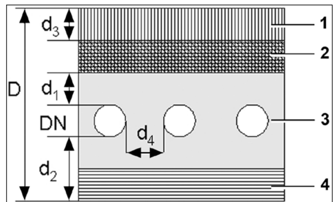
1 Estrich 2 Dämmung 3 Betonplatte mit Lüftungsrohr 4 Filigrandecke
