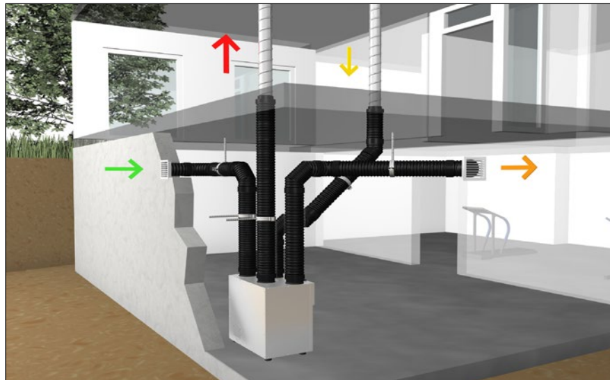
Außen- und Fortluftleitungen mit dem wärmegeprägten Lüftungsrohrsystem MAICOTherm.
