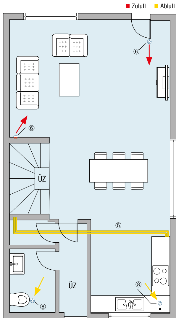
Erdgeschoss
