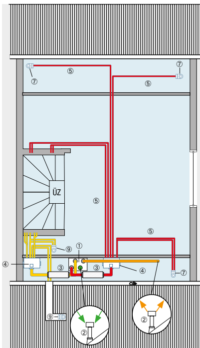
Dachgeschoss (DG)
