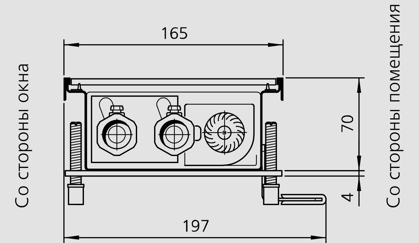
В разрезе (увеличенный), пример с поперечной решеткой
