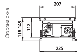
В разрезе (пример с рулонной решеткой)
